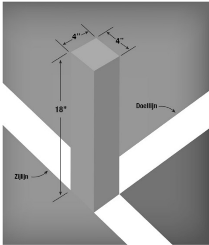
DETAIL VAN PYLON
