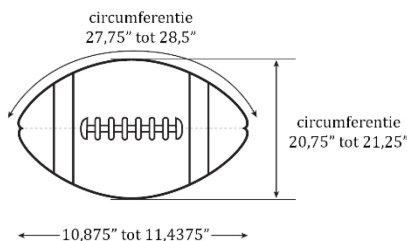
Diagram met de dwarsdoorsnede in de lengte van de standaardbal. De maximale en minimale afmetingen worden vermeld. Dit diagram staat in de regels om uniformiteit bij de fabricage te waarborgen.
